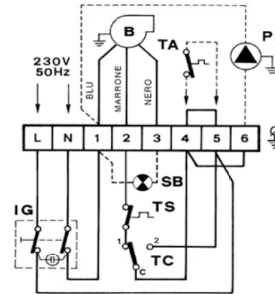
Рисунок 2. Электрическое подключение.
