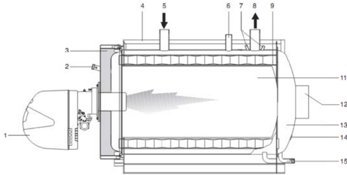
Рисунок 1. Описание котла.
